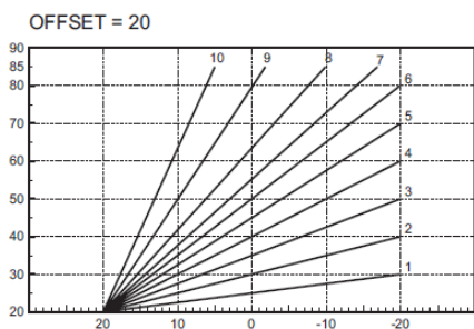
شکل (۱۰) مثالی از جابجایی نمودار جبران
